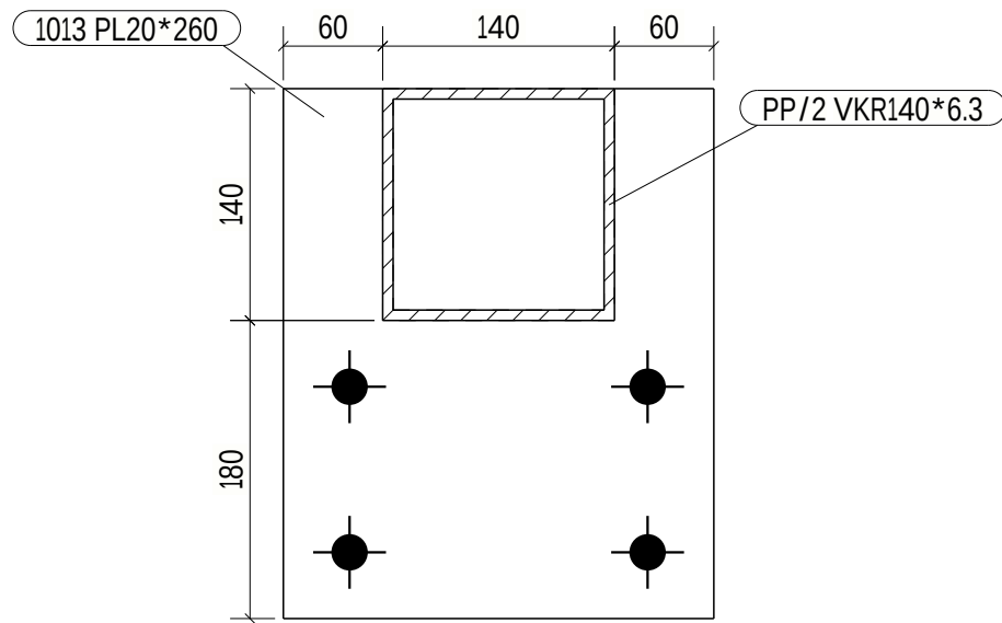
B - B 1:5
